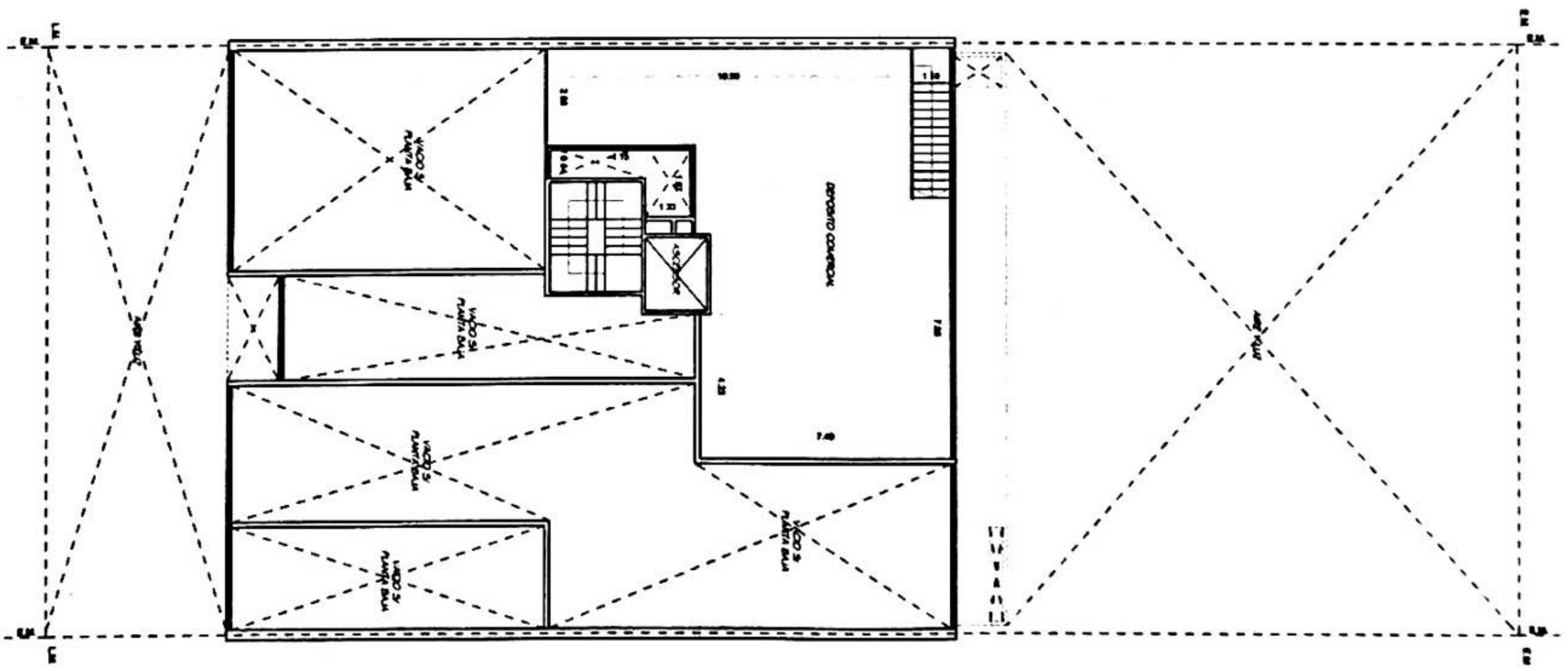
PLANTA ENTREPISO
