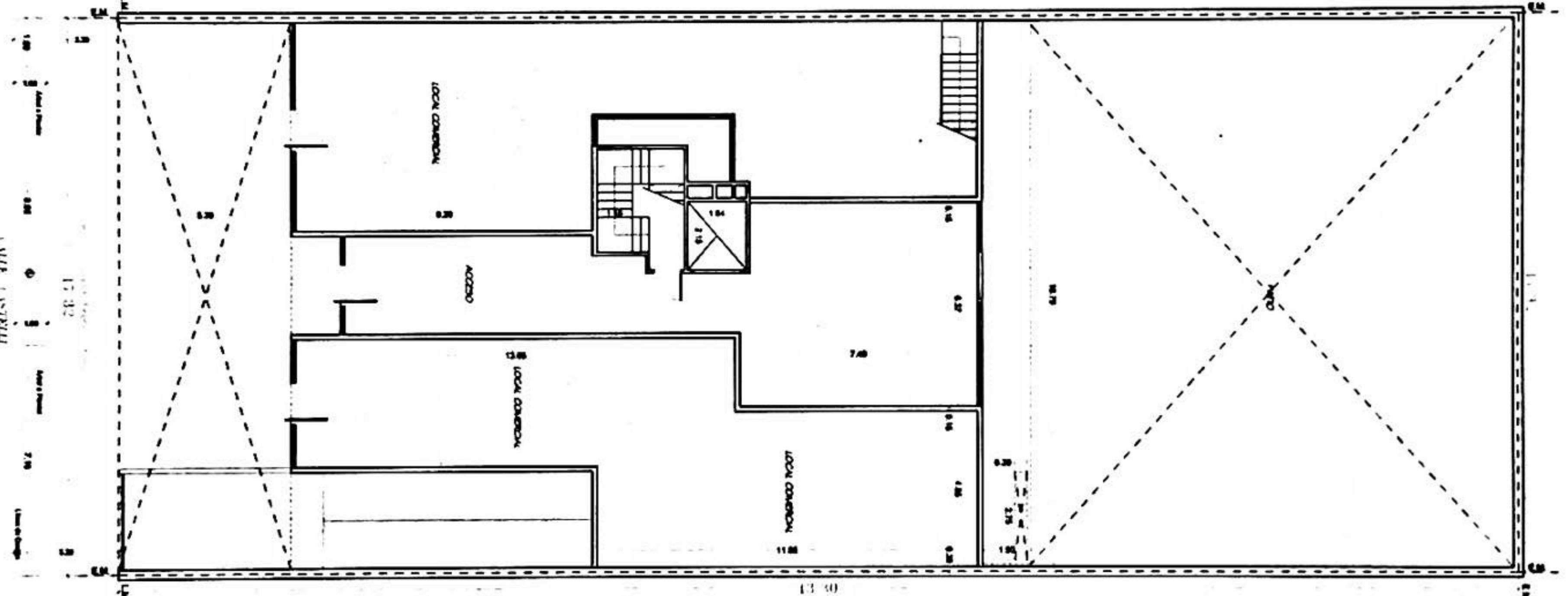
PLANTA BAJA
