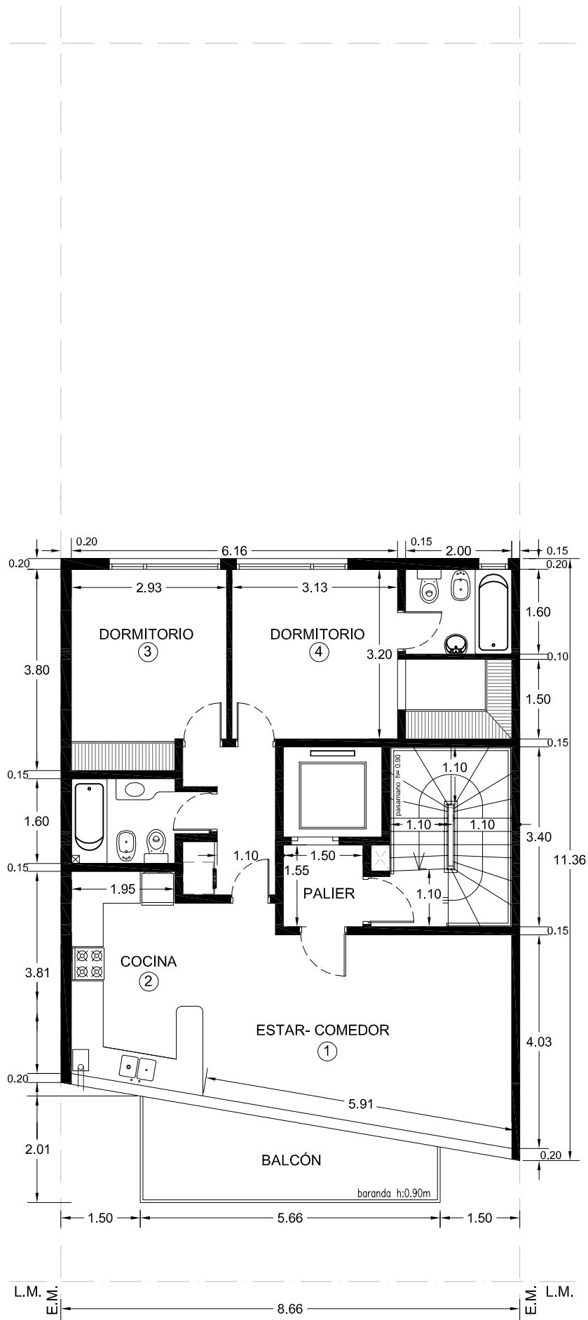
PLANTA TIPO 1º a 5º
